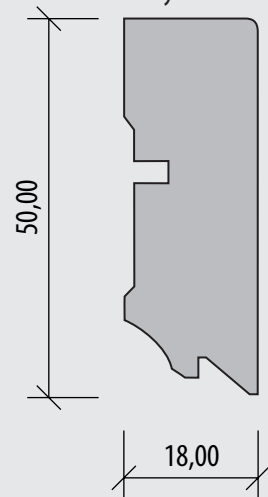
Lišty Hoco 634
