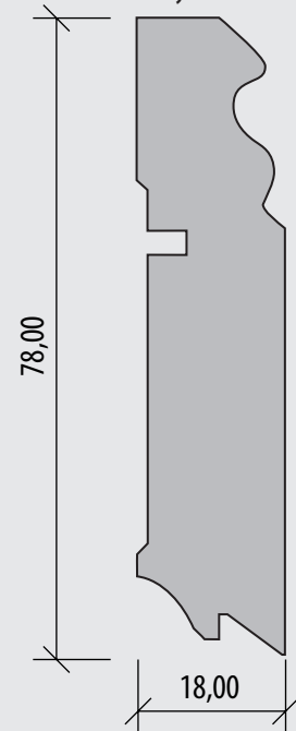
Lišty Hoco 626
