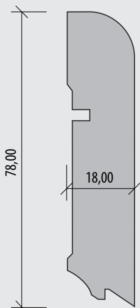
Lišty Hoco 606
