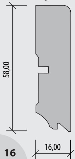
Lišty Hoco 631
