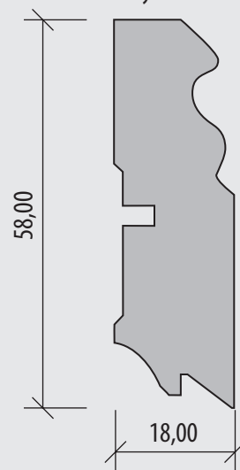
Lišty Hoco 624
